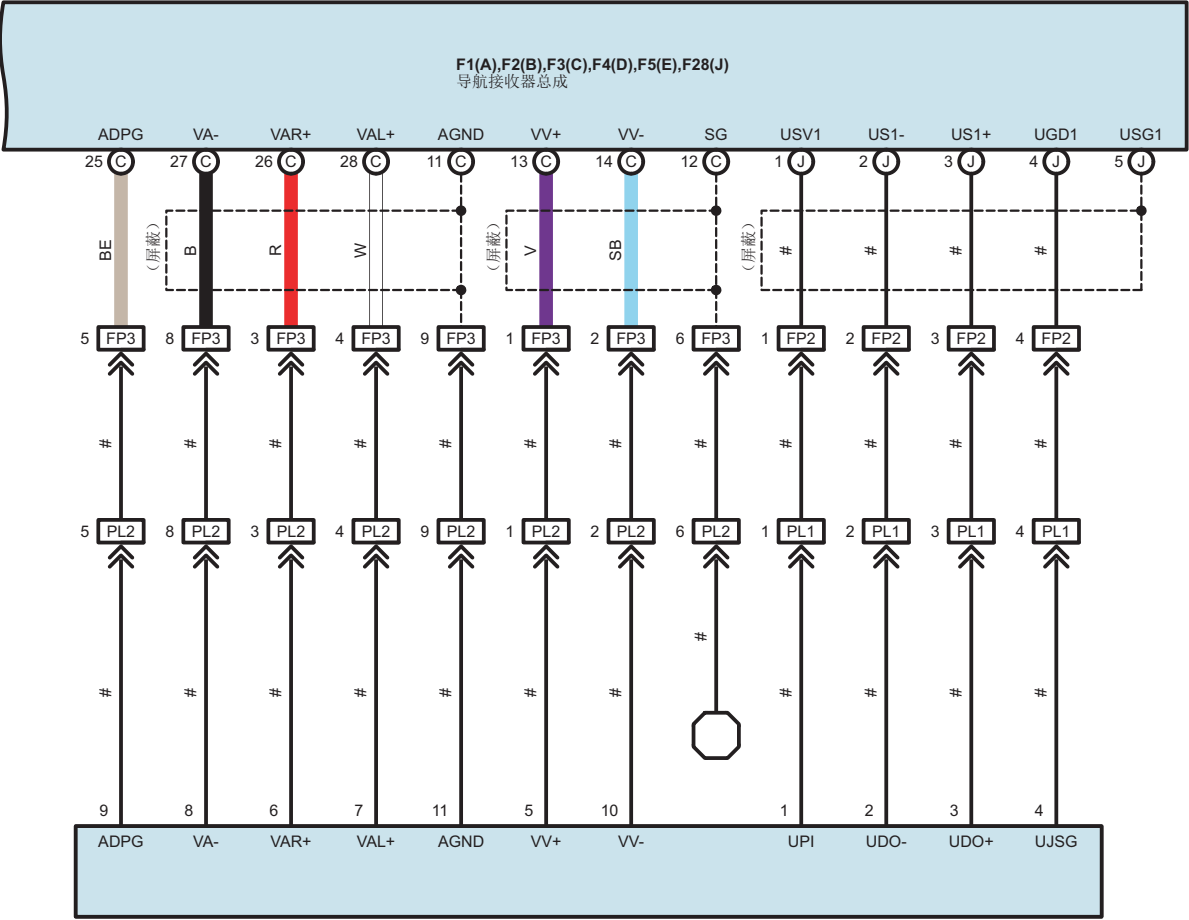
L36 1 号立体声插座适配器总成
